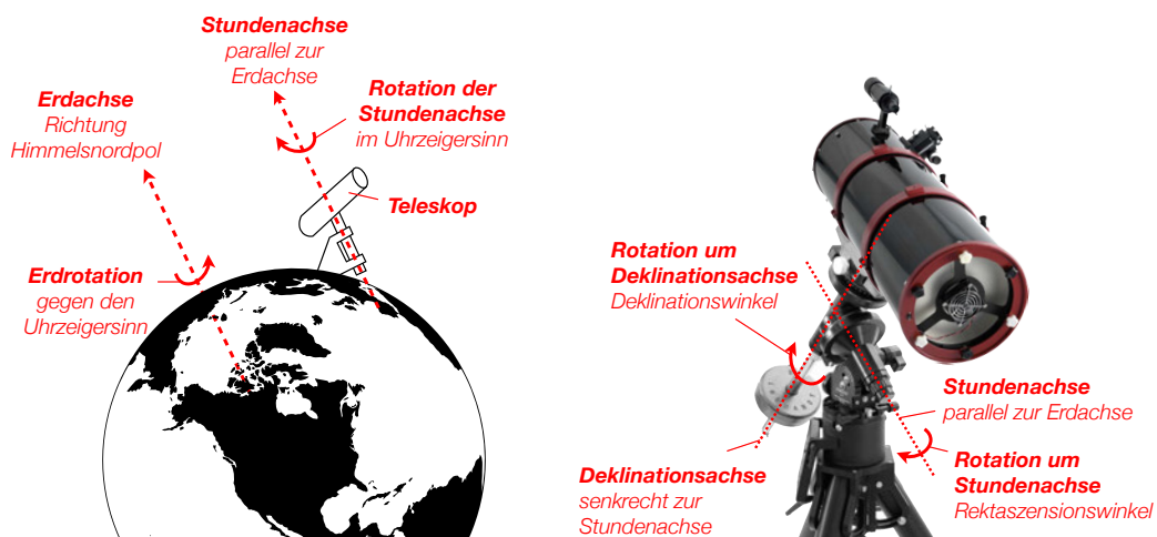
Abbildung 2: Prinzipskizze zur Idee der äquatorialen Montierung (links) und konkrete kommerzielle Umsetzung (rechts).
