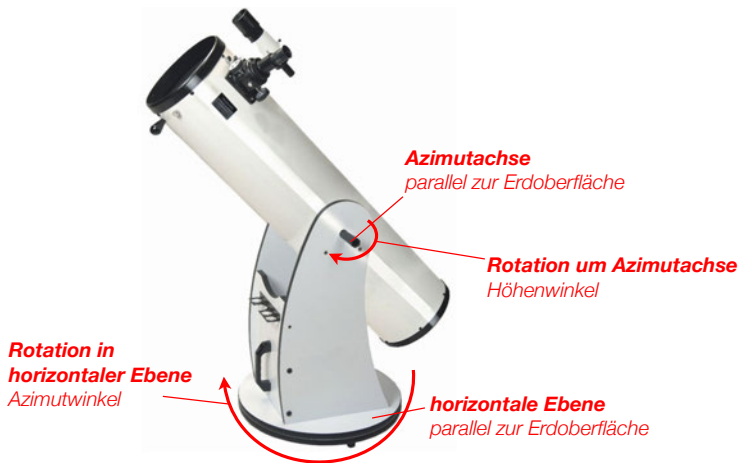
Abbildung 3: Kommerzielle Umsetzung einer azimutalen Montierung.
