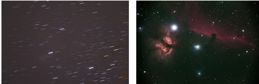
Abbildung 1: Pferdekopfnebel (IC 434) im Sternbild Orion. Links: 120s Belichtungszeit ohne Ausgleich der Erdrotation. Rechts: 120s Belichtungszeit mit Ausgleich der Erdrotation.
